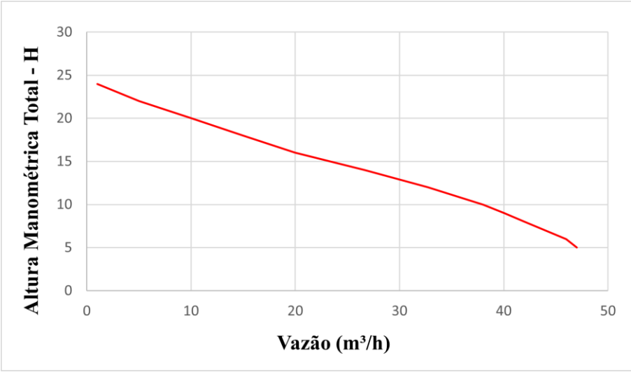
Figura 06 - Altura manométrica e vazão da bomba submersível modelo Lepono
