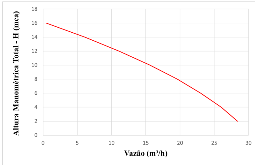
Figura 04 - Altura manométrica e vazão da bomba submersível modelo Lepono LSWm200CA
