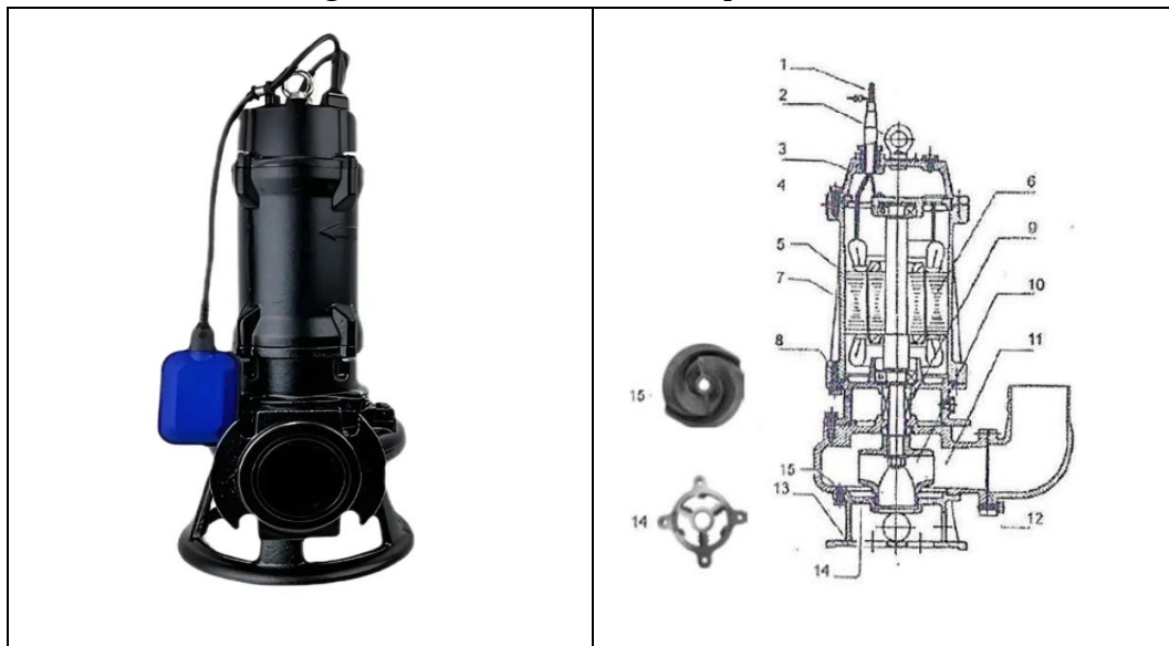
Figura 05 - Bomba modelo Lepono WQ25-15-22
