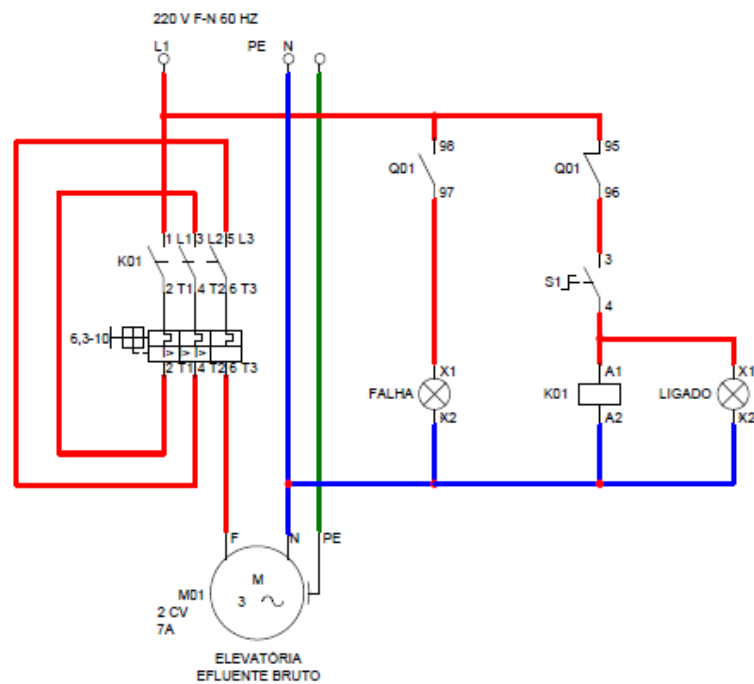
Figura 10 – Diagrama Elétrico modelo LSWm200CA (2,0 CV).
